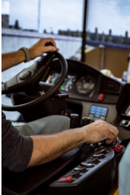
Detailansichten des Fahrsimulators – für ein echtes „Look & Feel“ wurden die originalen Komatsu Armaturen verwendet
